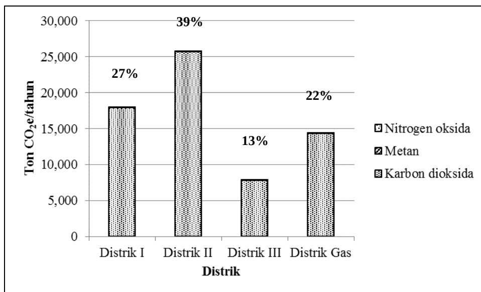
Gambar 2 Beban emisi pembakaran dari stationary device
