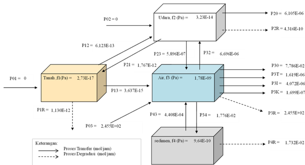
Gambar 4. Skema fugasitas pencemar DDT
